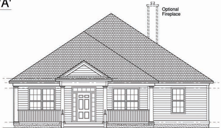
Elevation 'B'
